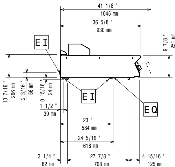
Zij aanzicht
