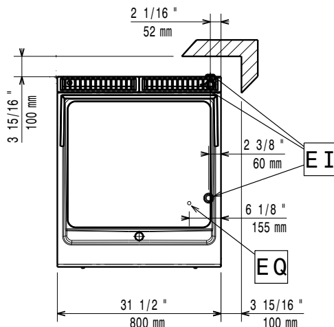
Boven aanzicht
